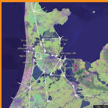
Een schematisch overzicht van de inlaatspunten en waterstromen (pijlen) en ook de inundatiestations (cirkels) voor de inundaties van de Stelling.
